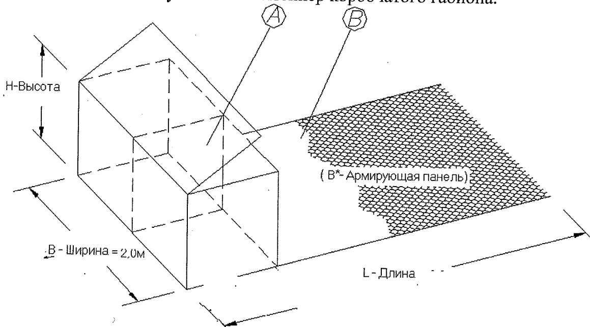
Рисунок Б.1 Контейнер коробчатого габиона.
