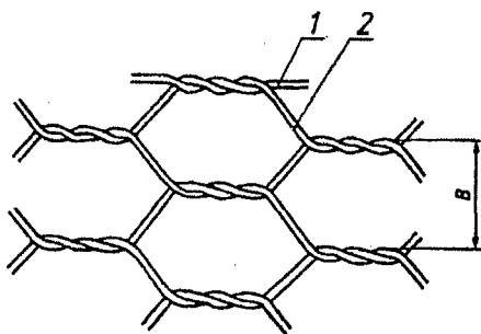
Рисунок 1. Схема шестиугольных ячеек сетки двойного кручения
