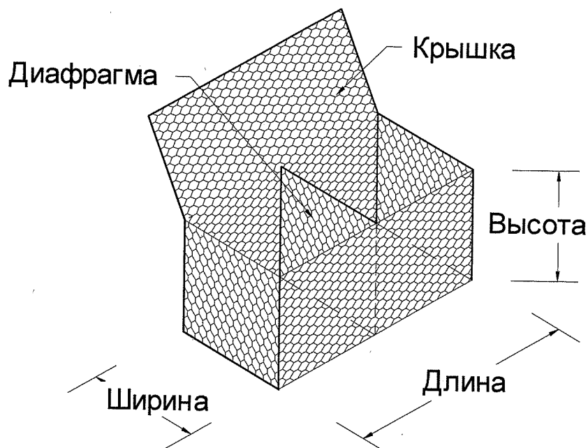
Рисунок Б.1 Контейнер коробчатого габиона.
