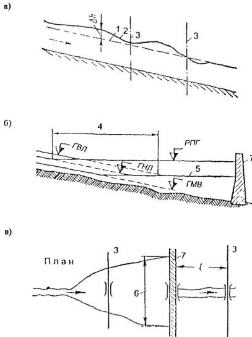
Рис. 3.10. Схемы уровней поверхностей воды:
