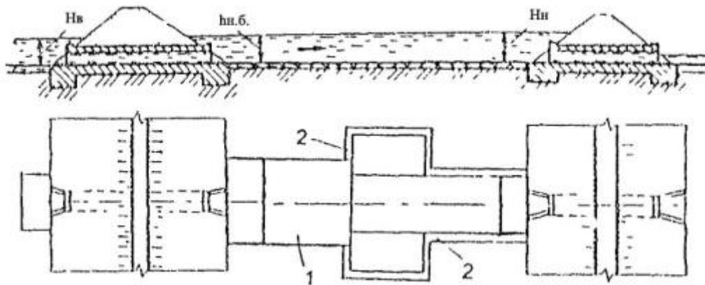
Рис.6.10. Схема противозрозионного сопряжения пространства между водопропускными трубами, расположенными на близлежащих дорогах или на раздельном дорожном полотне:
