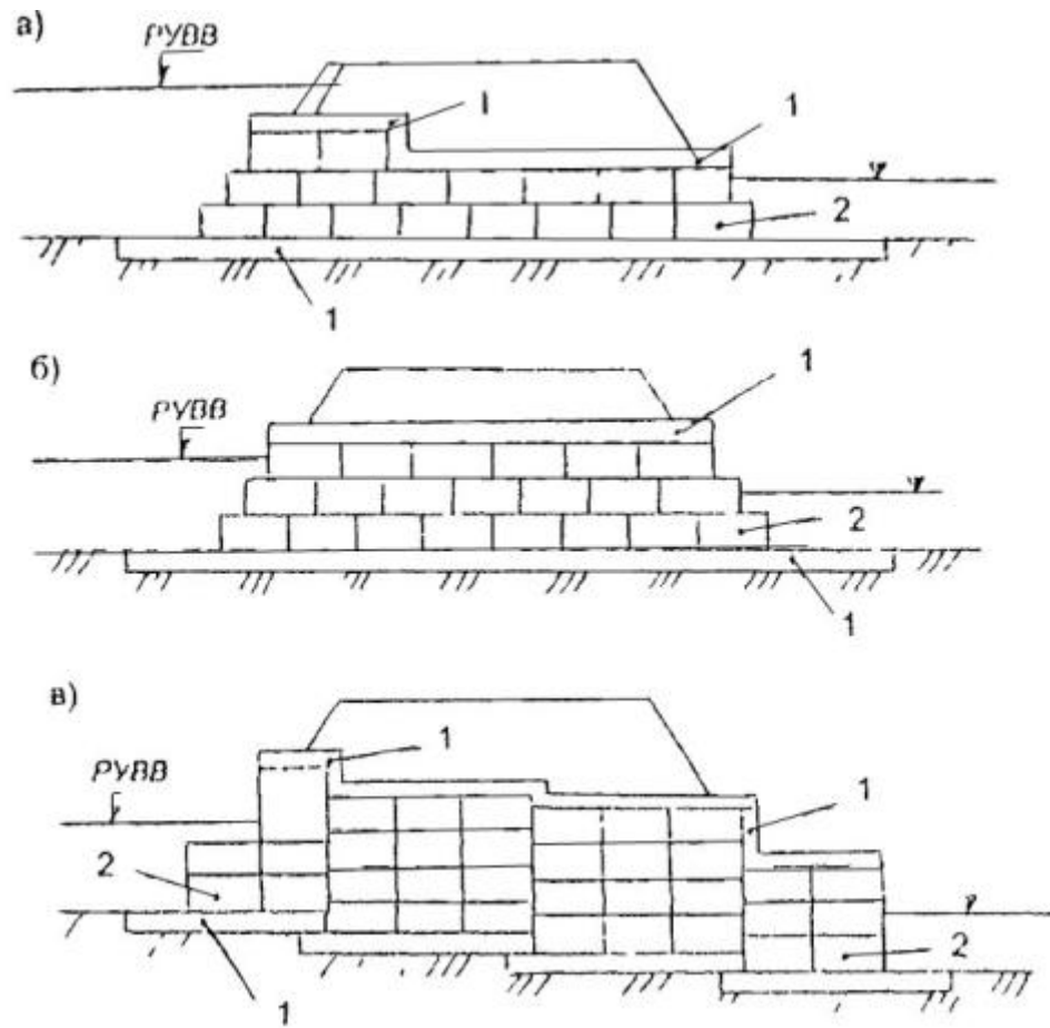
Рис. 7.6. Фильтрующие незатопляемые насыпи из коробчатых габионов:
