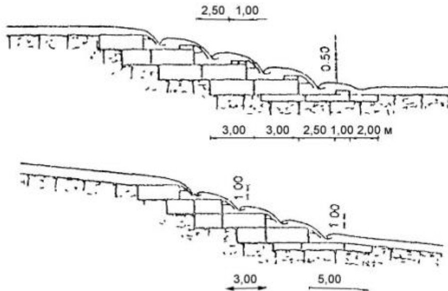
Рис. 7.2 Схема устройства многоступенчатых габионных перепадов в нижнем бьефе переливаемых насыпей и сооружений.
