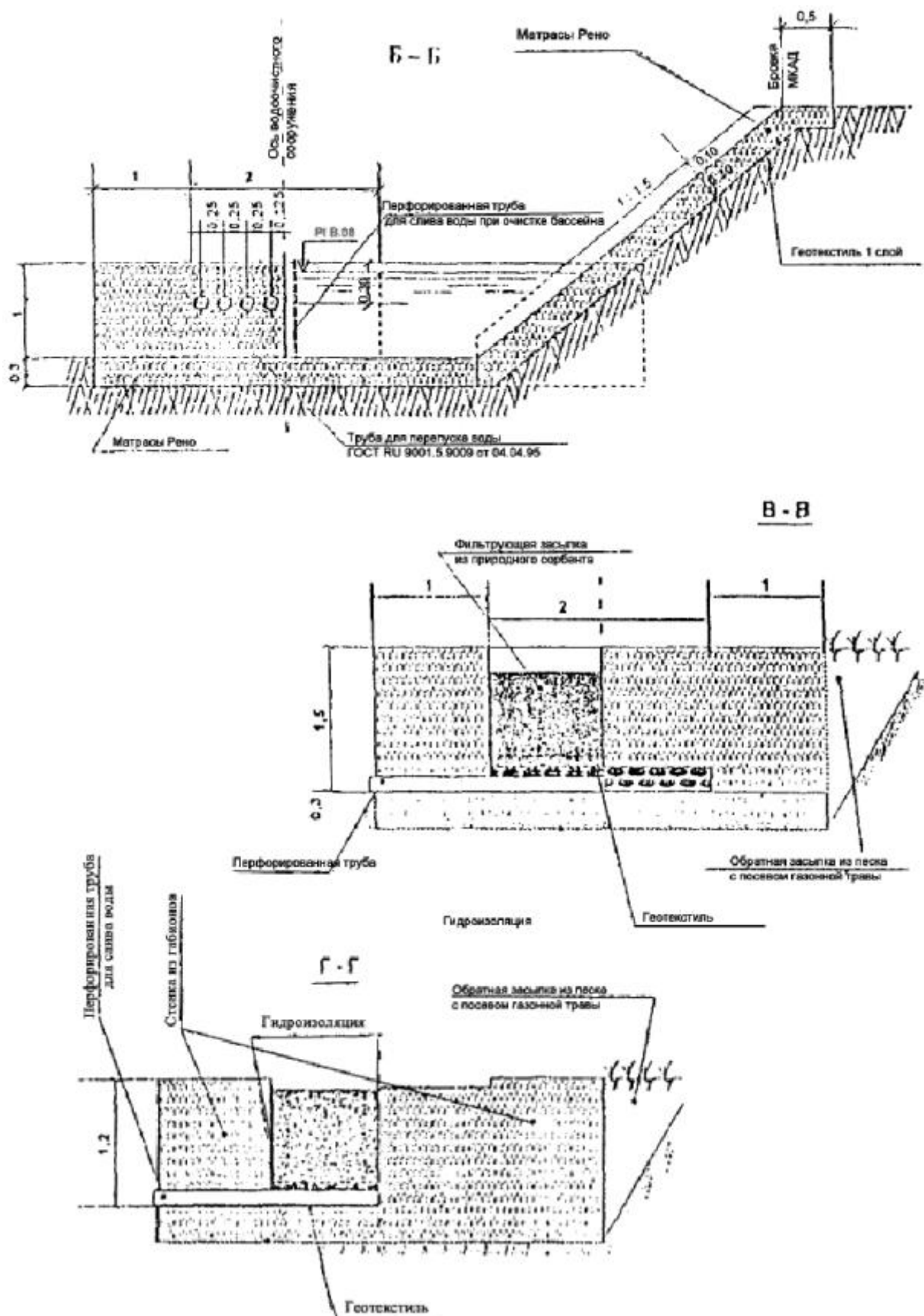
Рис. 6.27. Элементы габионного очистного сооружения (рис. 6.26.).
