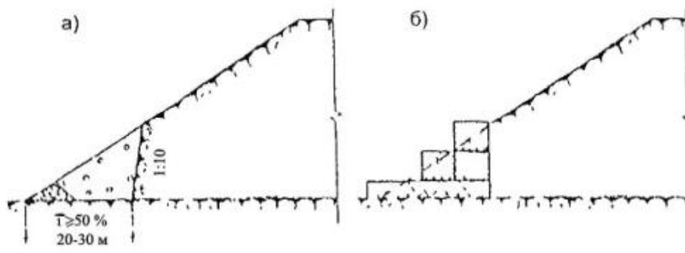
Рис.5.7. Дренажные шпory в откосе:
