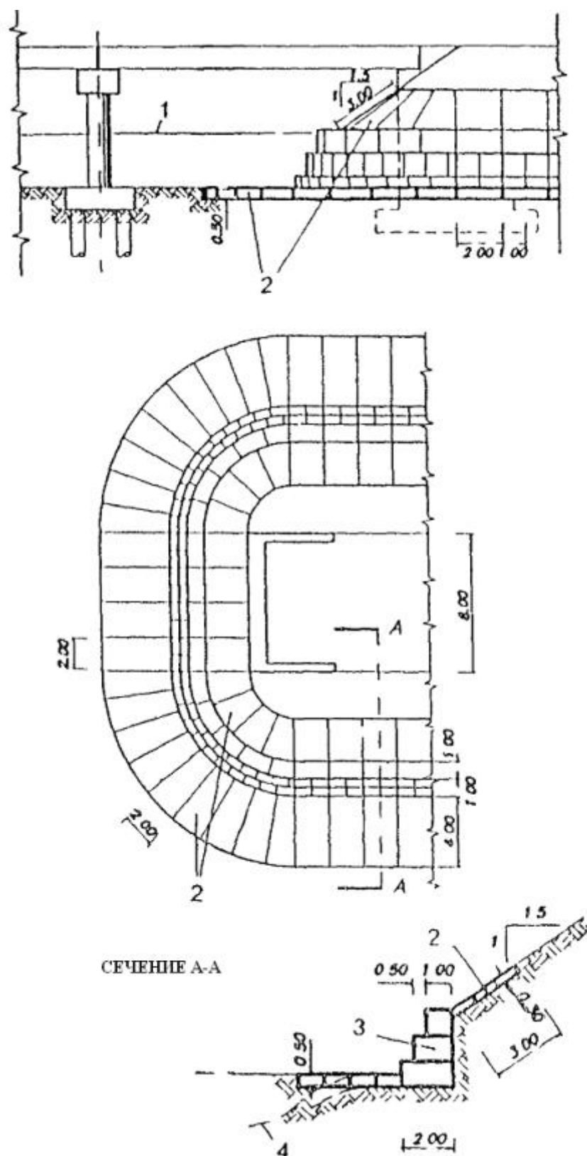
Рис. 4.5. Схема габионного укрепления подмостовых конусов, стесняемых пролеты мостов с размываемыми руслами:
