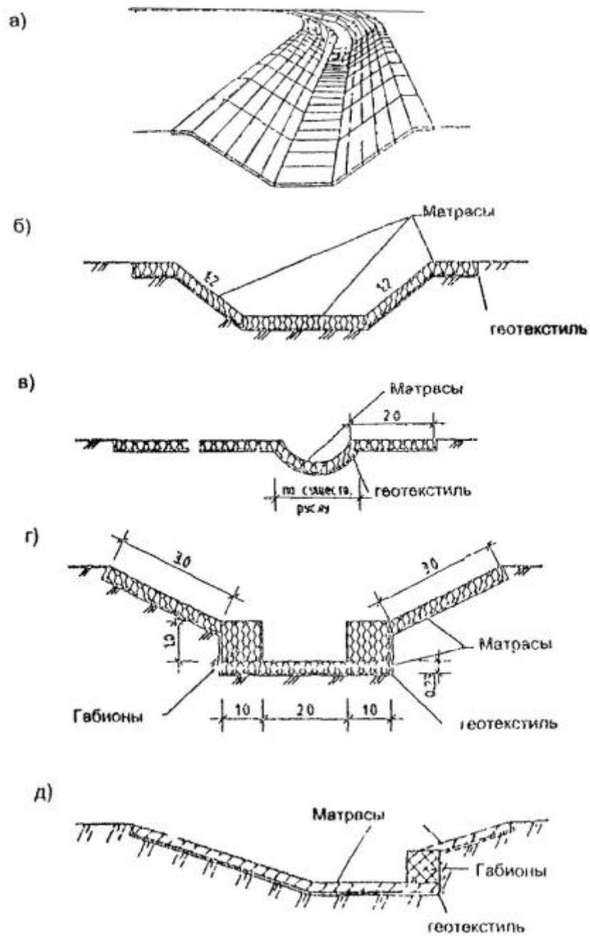
Рис. 6.21. Схемы габбионных укреплений водоотводных канав, резервов и кюветов.
