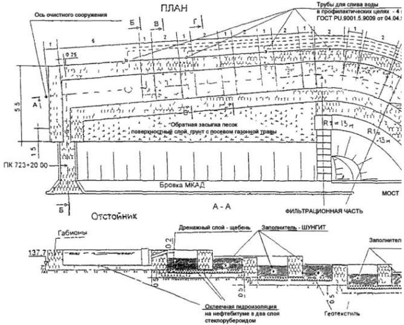
Рис. 6.26. Габрионное очистное сооружение.
