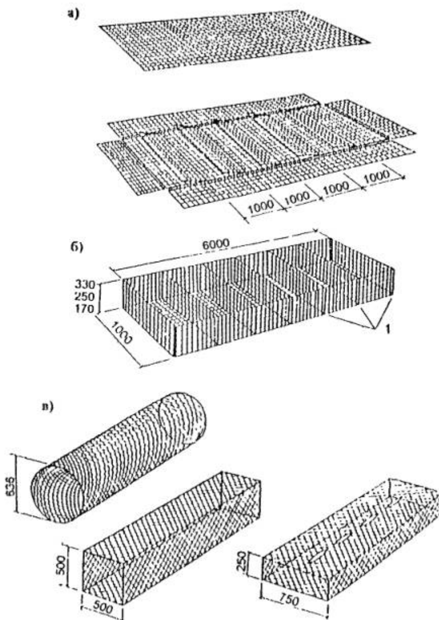
Рис. 2.27. Каркасы габионов:
