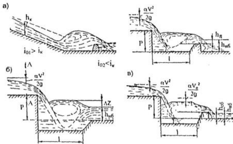
Рис.6.18. Формы кривых свободной поверхности водных потоков в водобойных устройствах( г ):
