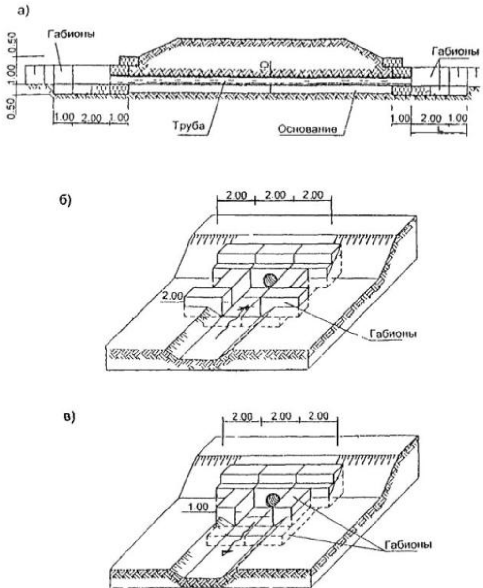
Рис. 6.4. Схемы возможных габийонных укреплений верхнего и нижнего бьефов круглых водопускных труб.
