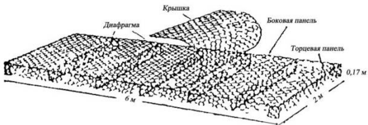
Рис. 2.8. Схема матрасно-тюфячного арматурного каркаса и его элементов в сборке.
