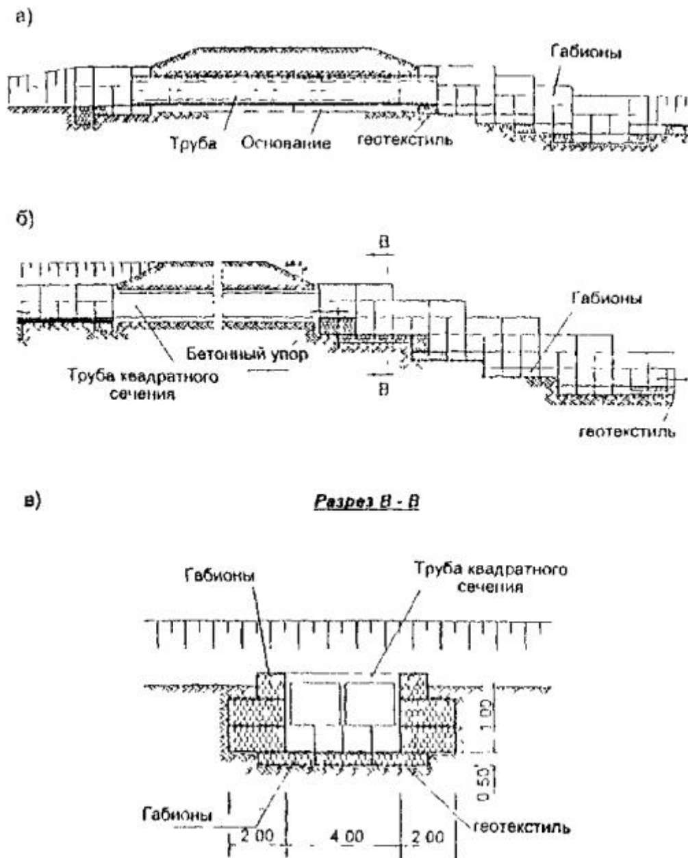
Рис. 6.13. Схемы возможных габйонных укреплений входных и выходных участков водопропускных труб с водобойными устройствами.
