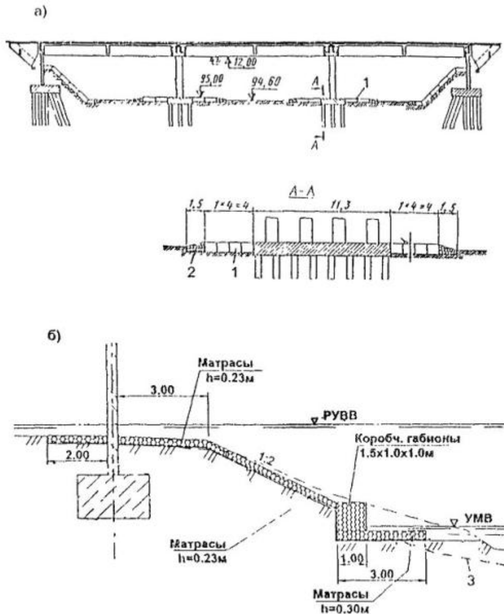
Рис. 4.8. Схемы габионных укрепений опор мостов при возможности возникновения их подмыва:
