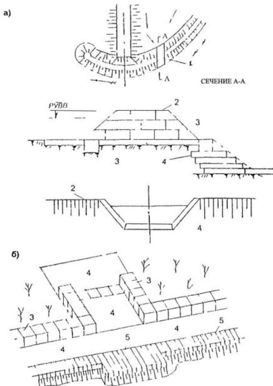
Рис. 4.28. Противоэрозионные габионные водосливы:
