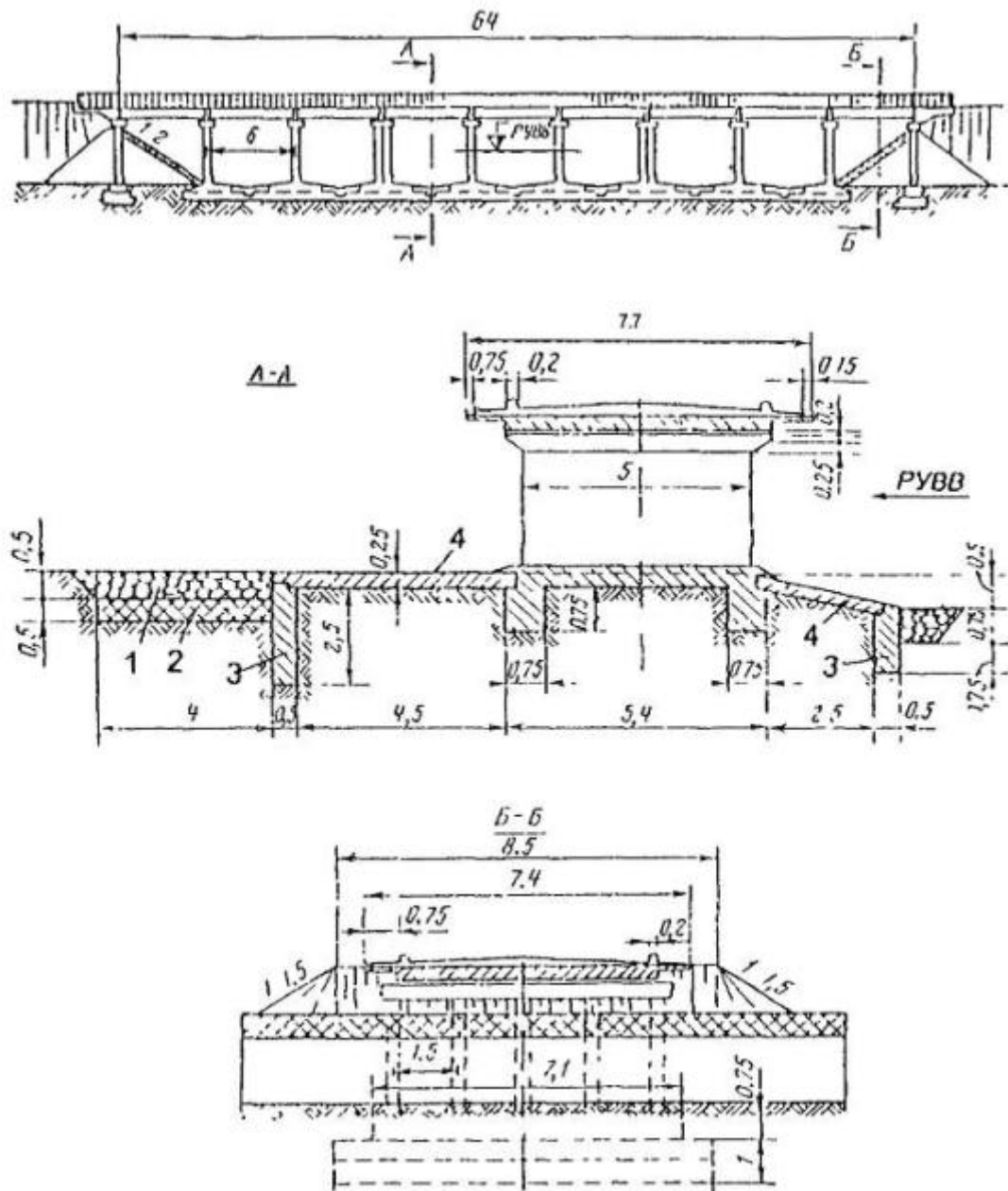
Рис. 4.13. Конструктивная схема моста с укрепленным руслом не предгорной реке:
