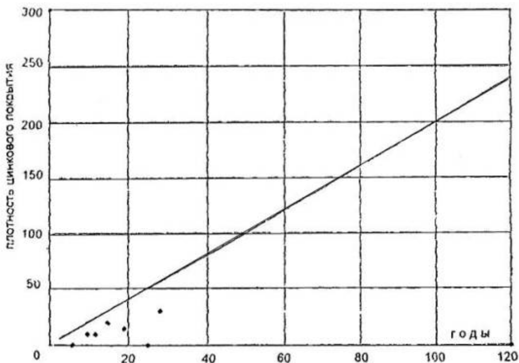
Рис. 2.13. Фактические значения срока службы ПВХ покрытия оцинкованных каркасов габионов на 7 эксплуатиремых зарубежных объектах.
