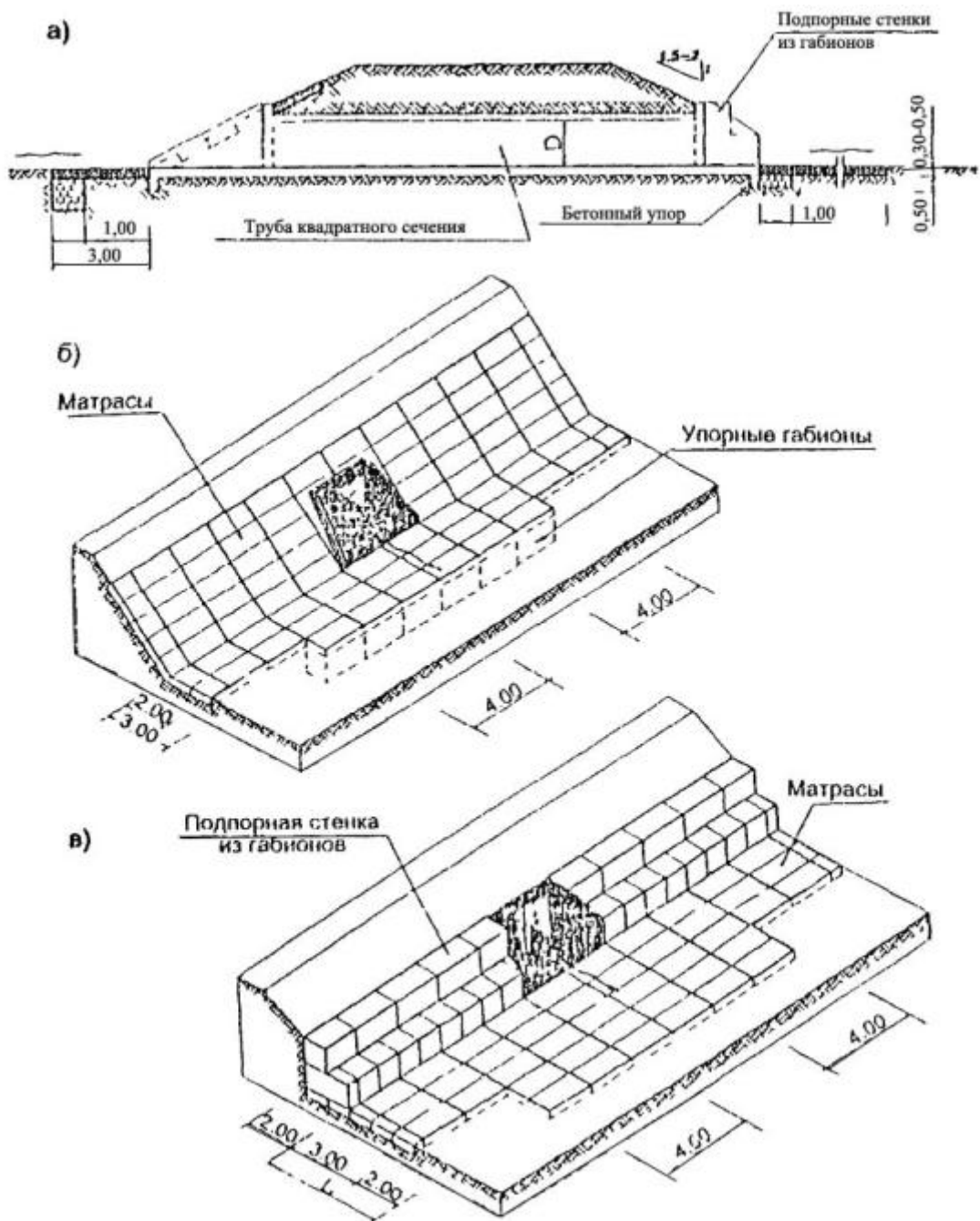
Рис. 6.6. Схемы возможных габионных укреплений верхнего и нижнего бьефов прямоугольных водопропускных труб.
