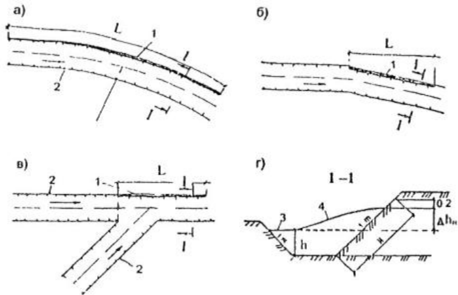
Рис. 6.22. Схемы к определению планово-высотных границ габионных укреплений водоотводных канав при искривлении движения водных потоков:
