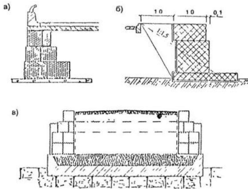
Рис. 5.3. Схемы конструктивных решений по замене откосных частей земляного полотна габийонными подпорно-удерживающими сооружениями.
