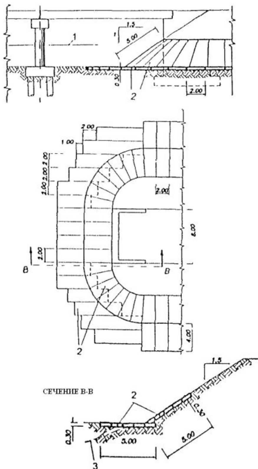
Рис. 4.4. Схема габионного укрепления подмостовых конусов, свободно размещаемых в пролетах мостов с размываемыми руслами:
