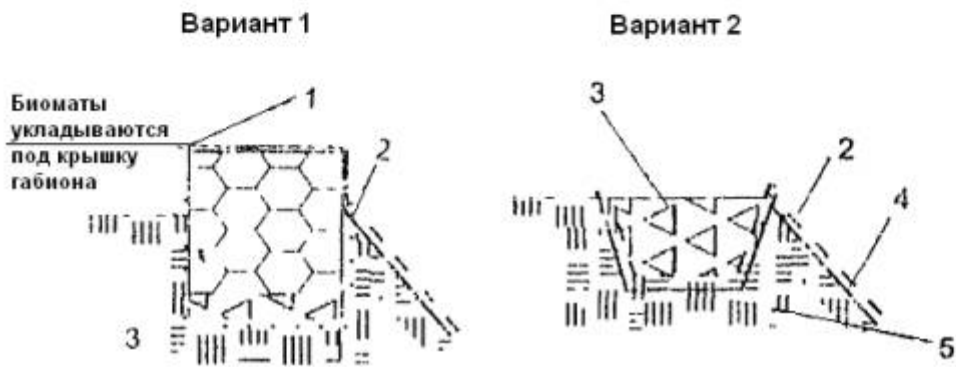
Рис. 3.3. Схема крепления откосов с использованием биоматов и коробчатых габионов:
