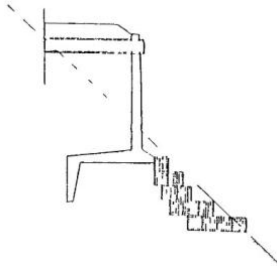
Рис.5.2. Схема габийонной конструкции для защиты фундаментов галлерей.
