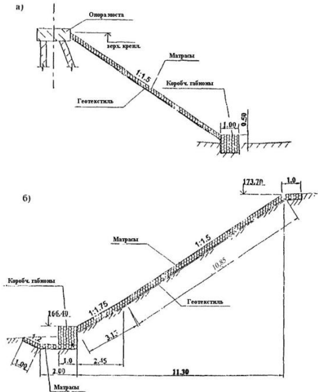
Рис. 3.6. Схемы укрепления неподтопляемых откосов габионными конструкциями:
